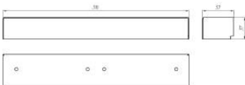
Крышка BS-KR-1
